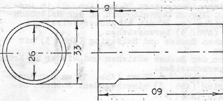
Reduzierbuchse 37 kW
