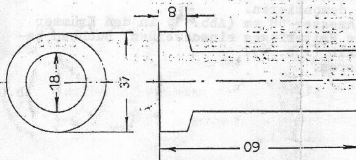
Reduzierbuchse 20 kW
